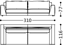
01DNIC1 (1DNIECASXP - 1DNIECADXP) 02DNIC1 (2DNIECASXP - 2DNIECADXP)
