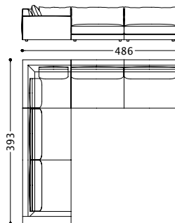
01DNIC34 (1DNIEGASXP - 1DNIEAP - 1DNIECA1P) 02DNIC34 (2DNIEGASXP - 2DNIEAP - 2DNIECA1P)
