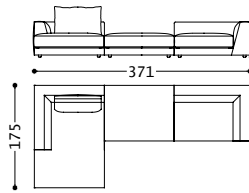
01DNIC26 (1DNIEBBDX - 1DNIEB - 1DNIEBBSXP) 02DNIC26 (2DNIEBBDX - 2DNIEB - 2DNIEBBSXP)
